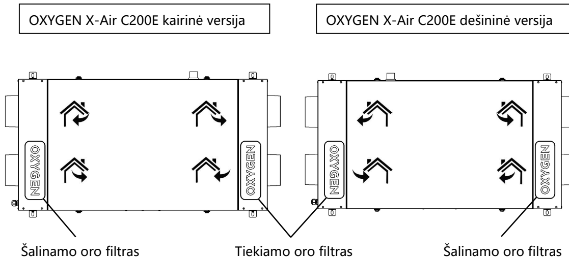
Pav. 10. Vėdinimo įrenginio filtrai
