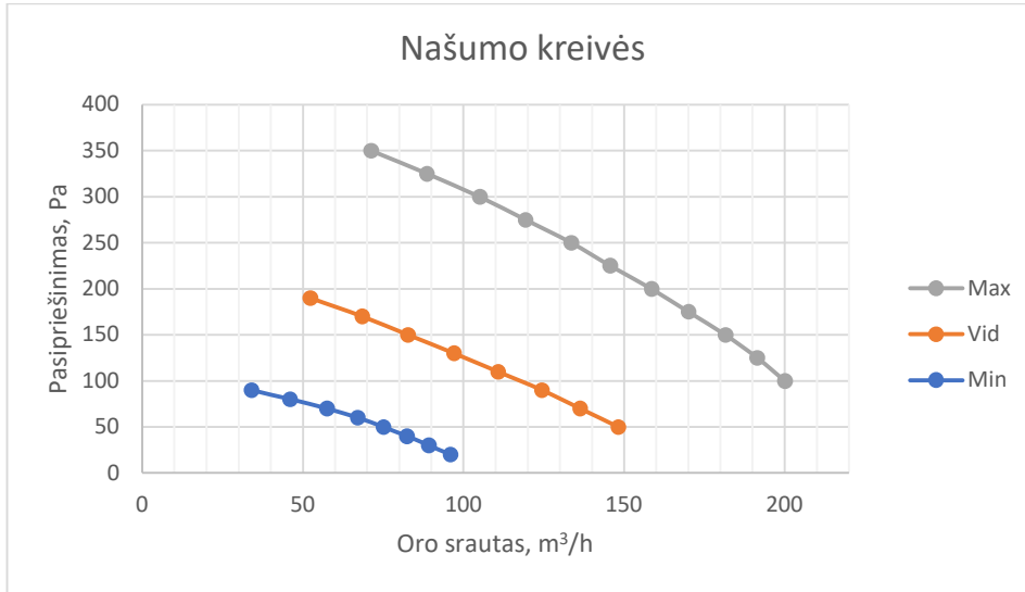
Graf. 1 Vėdinimo galios priklausomybė nuo įrengtos vėdinimo sistemos pasipriešinimo
