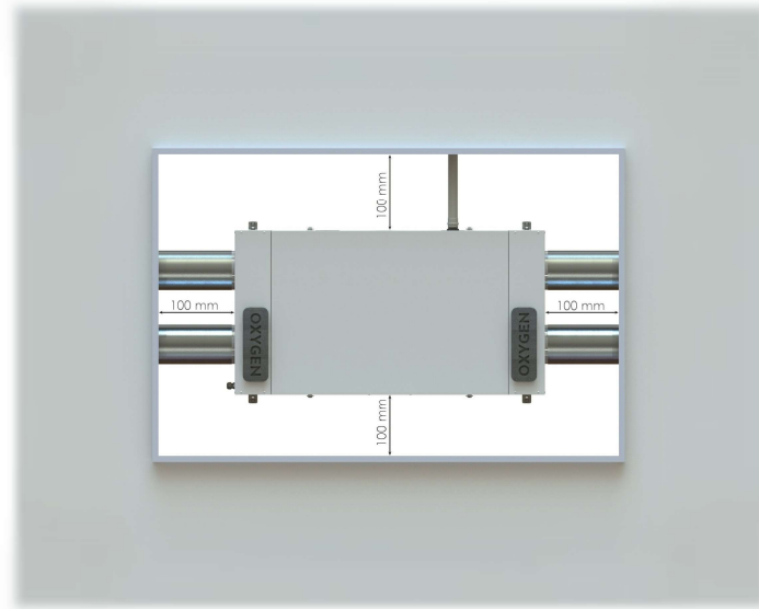
Pav. 4. Priežiūros bei aptarnavimo liukas
